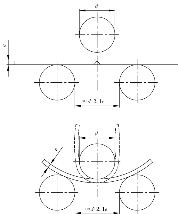
图6 对接接头弯曲试验
